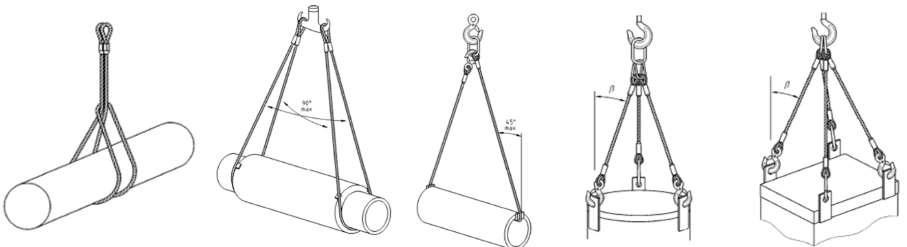
Imágenes extraídas de la norma UNE-EN 13414. Eslingas de cable de acero. Seguridad
